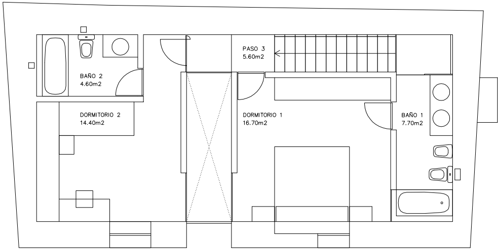
PLANTA PRIMERA TOTAL SUP. UTIL 49.00 m² TOTAL SUP. CONST. 70.60 m²
